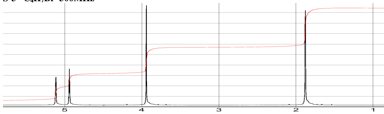
S-3 C 4 H 7 Br 300MHz
