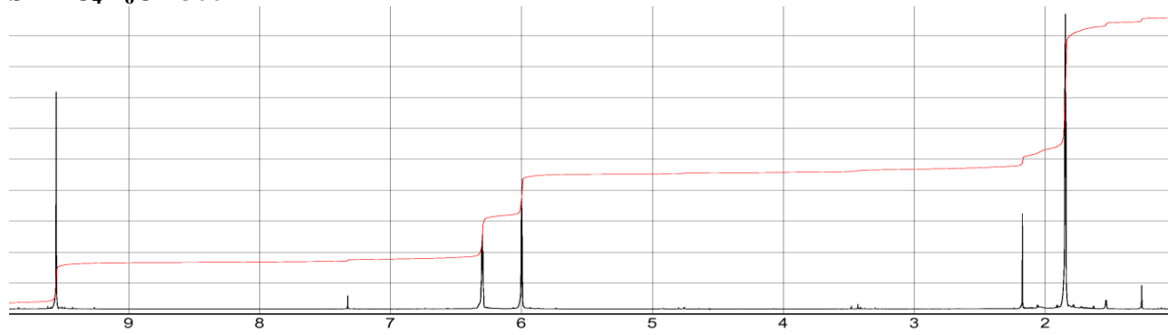
S-4 C 4 H 6 O 300MHz
