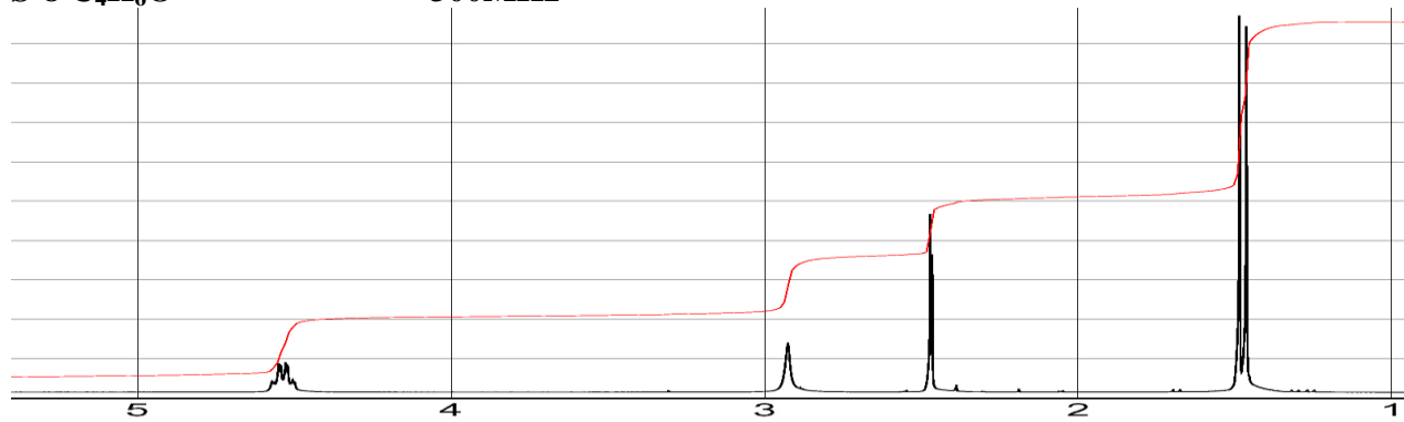
S-8 C 4 H 6 O 300MHz
