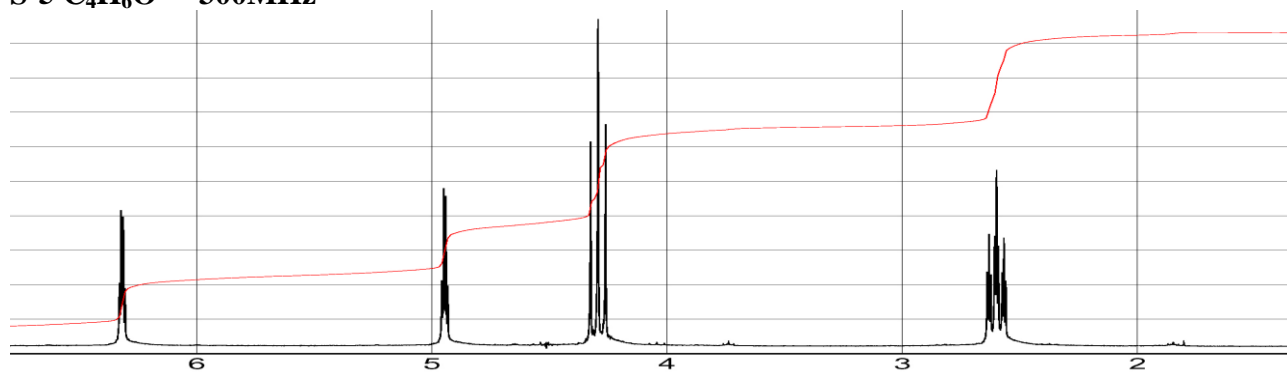
S-6 C 5 H 9 Br 300MHz
