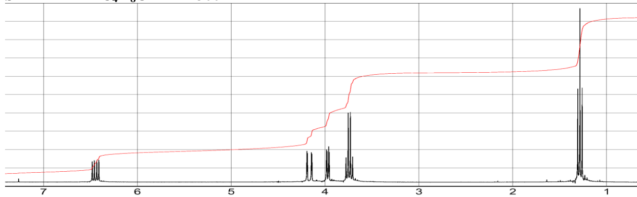
S-1 C 4 H 8 O 300MHz
