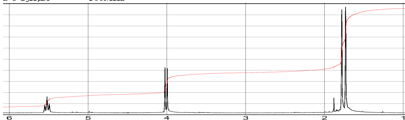
S-6 C 5 H 9 Br 300MHz
