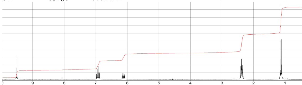
S-2 C 5 H 8 O 300MHz
