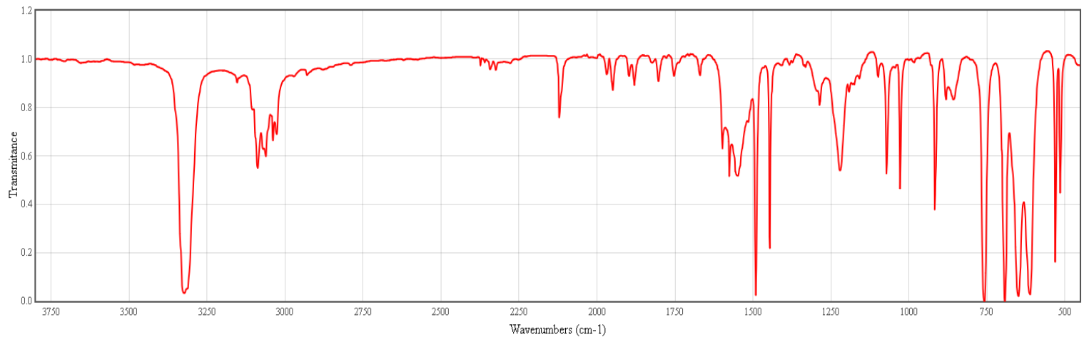
IR-A2 C 7 H 6 O 2
