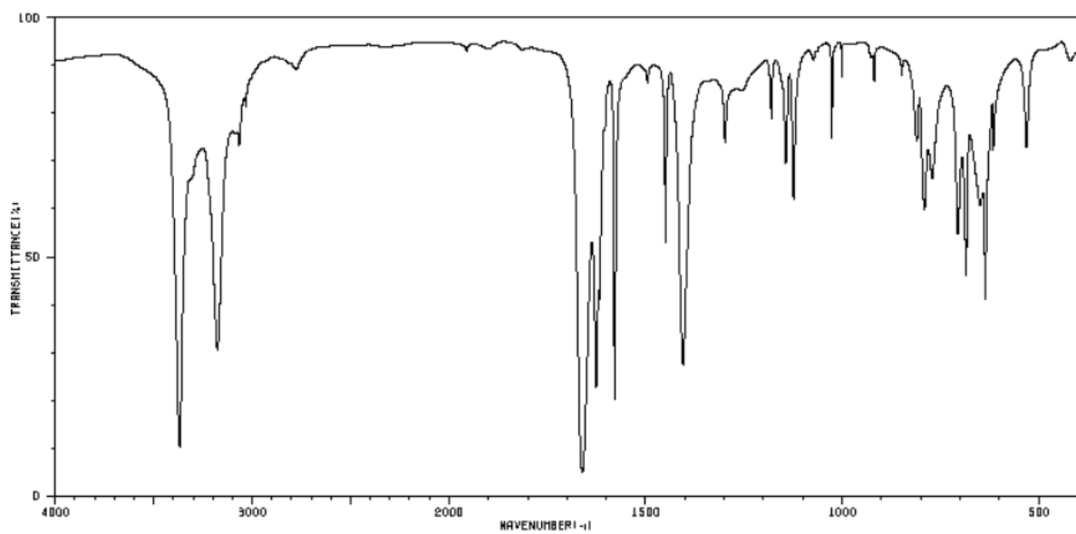
IR-A3 C 7 H 7 NO
